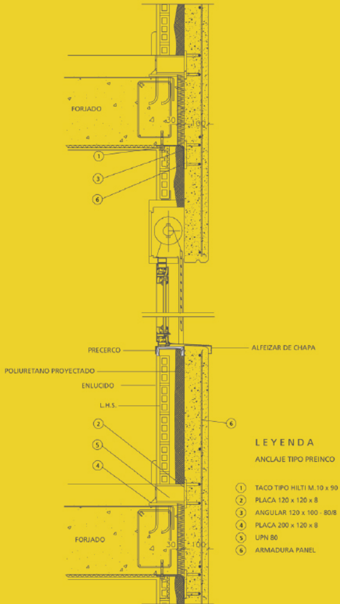
DETALLE FACHADA POR VENTANA TIPO PANEL ARQUITECTÓNICO
