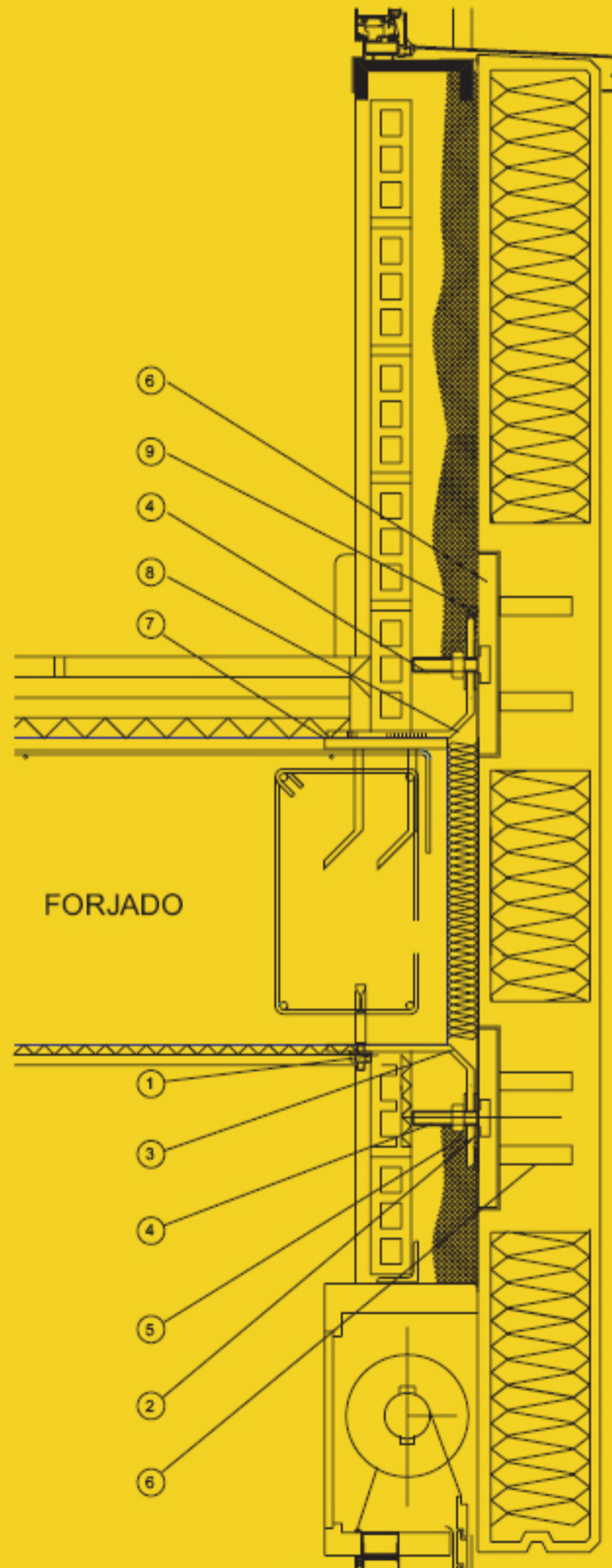
DETALLE PANEL ANTEPECHO TIPO SANDWICH
